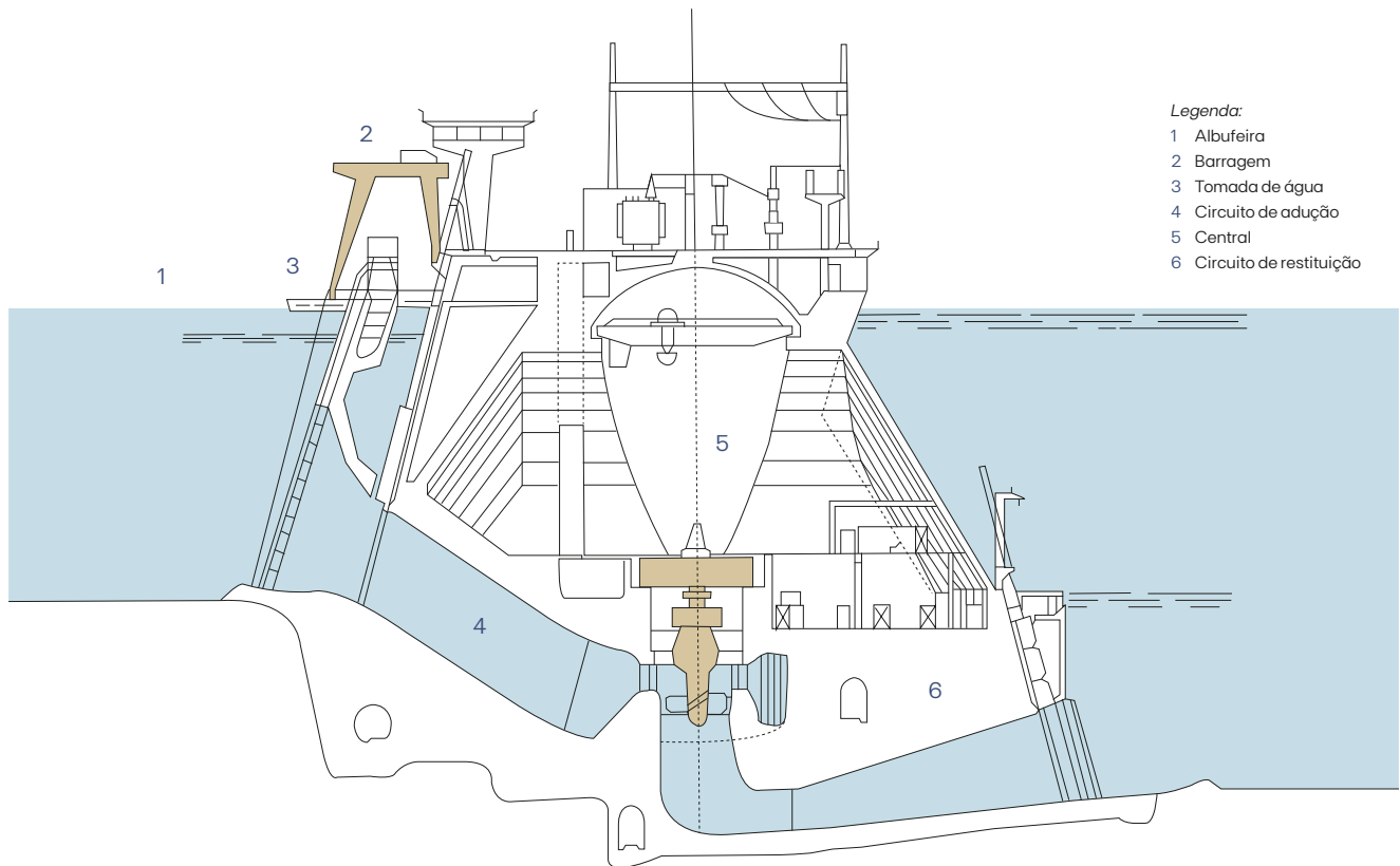
Circuito hidráulico
