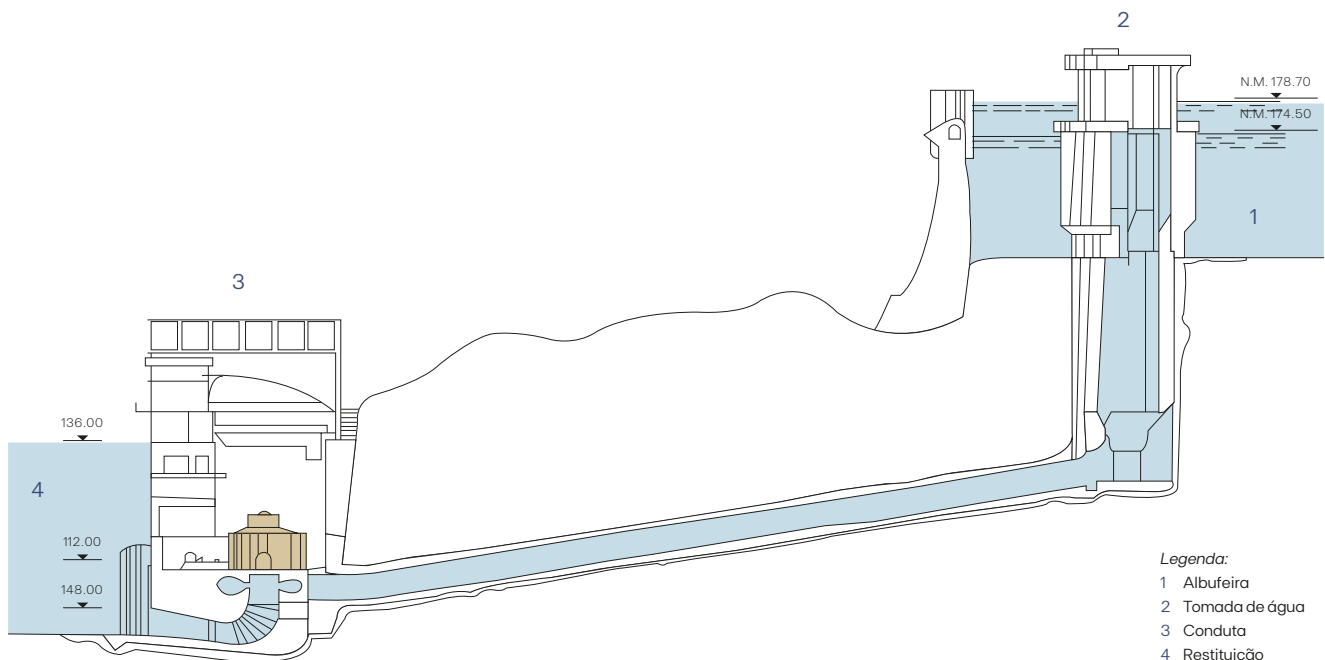
Circuito hidráulico
