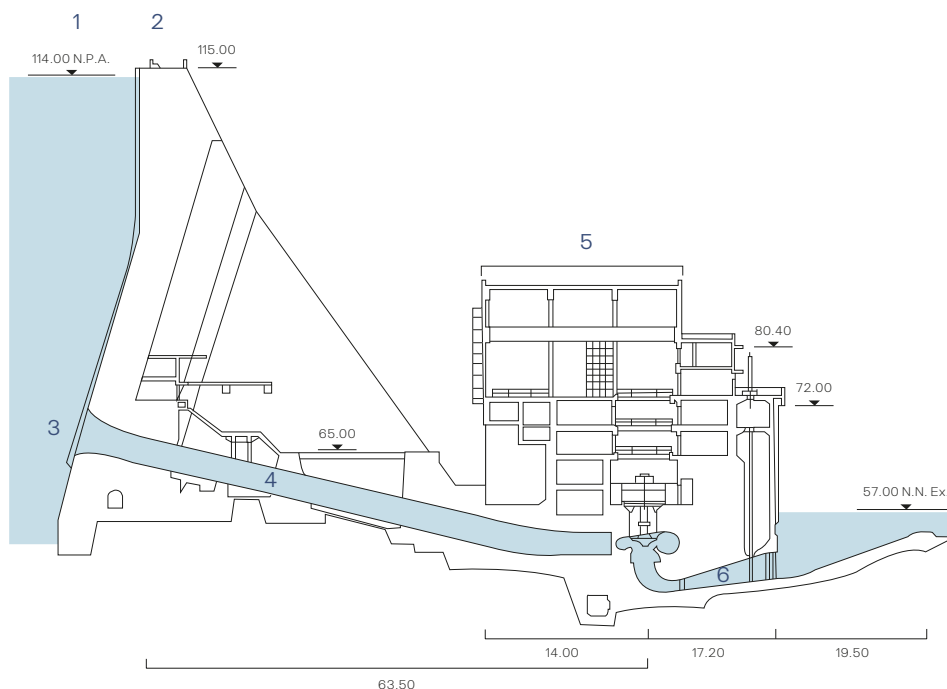
Circuito hidráulico do aproveitamento hidroelétrico da Pracana
