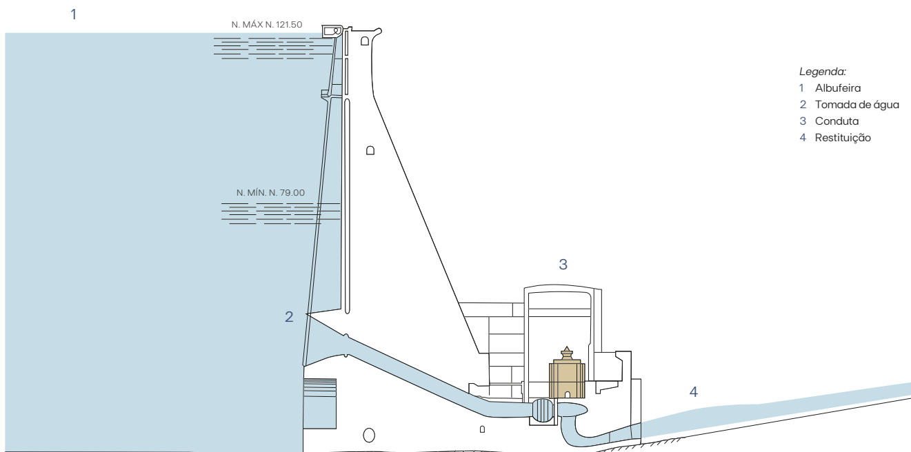
Circuito hidráulico
